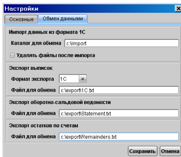
Рис. 3. Окно Настройки . Закладка Обмен данными
